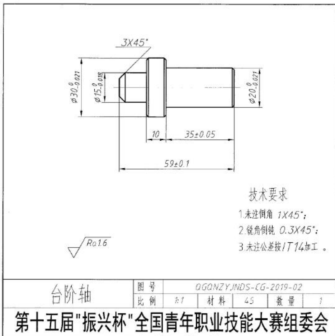
图 2. 台阶轴
